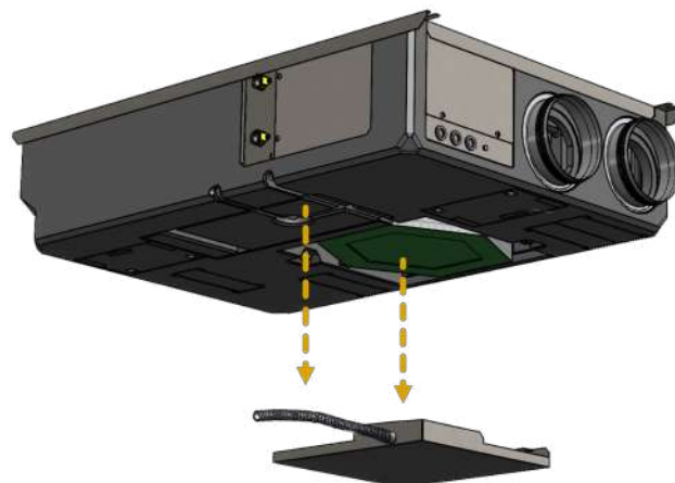
Passaggio #6: rimuovere dalla sede il tubo di scarico e, successivamente, rimuovere la vaschetta scarico condensa recuperatore (non scollegare il tubo, deve rimanere collegato come nell'immagine)
