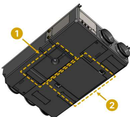
Passaggio #4: localizzare le vaschette condensa (2) e del recuperatore (1)
