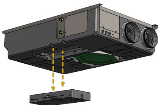
Passaggio #5: rimuovere dalla sede il tubo di scarico e, successivamente, rimuovere la vaschetta scarico condensa (non scollegare il tubo, deve rimanere collegato come nell'immagine)
