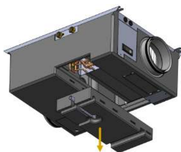
Passaggio 3: rimozione della vaschetta
