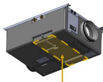
Passaggio 1: Localizzazione della vaschetta di raccolta della condensa e drenaggio della condensa
