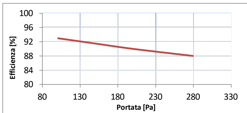
Curva di prestazione RDE 020
