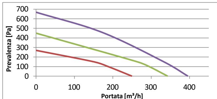
Curva portata – prevalenza RDE 035
